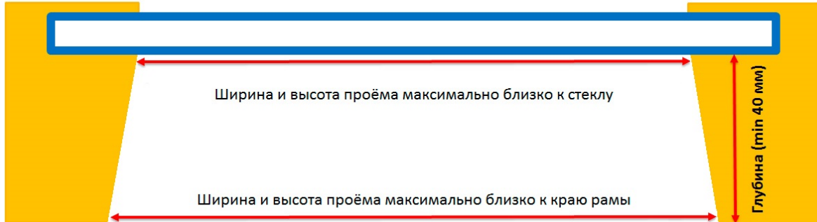
Оконная рама в разрезе. Вид сверху
